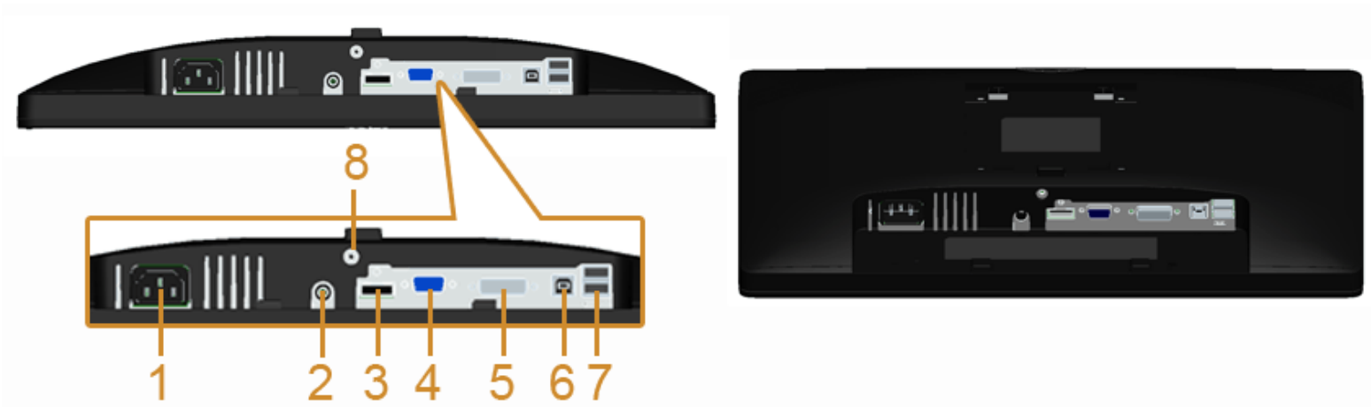
Ansicht von unten ohne Monitor-Standfuß
